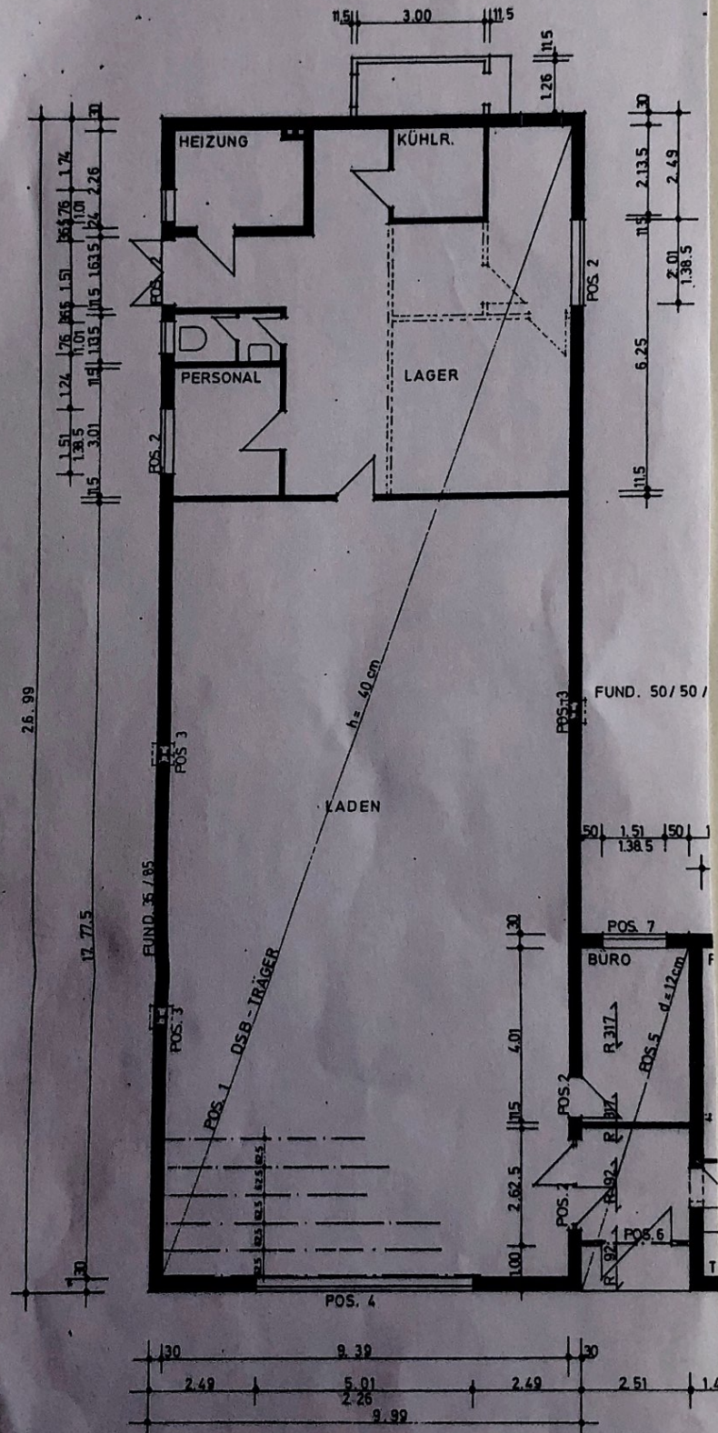
ERDGESCHOSSGRUNDRISS
